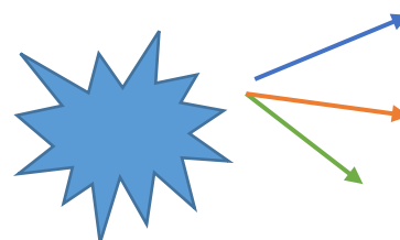
Точка бифуркации
